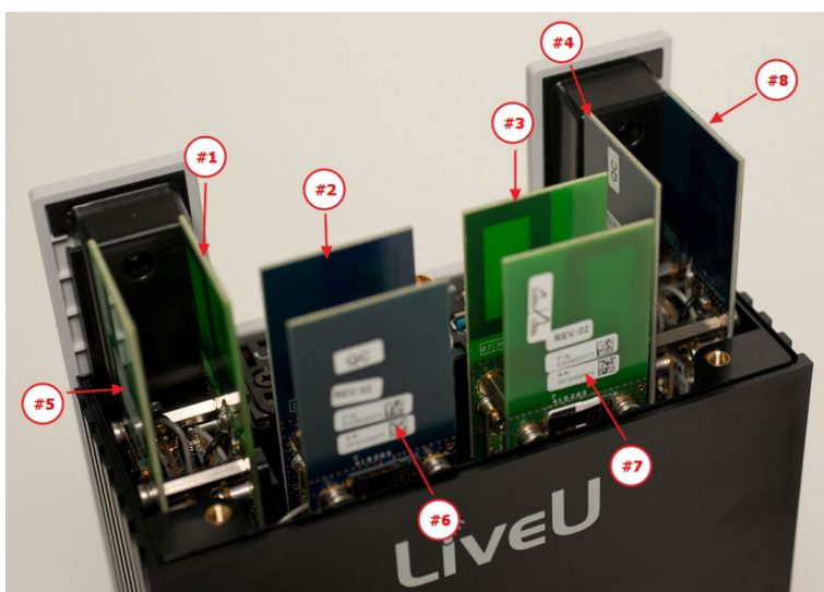
4. ábra: az LU500 modemjeinek számozása
